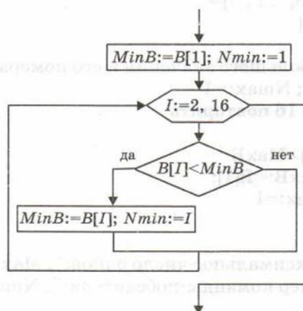
Рис. 2.14. Фрагмент блок-схемы — поиск минимального элемента
