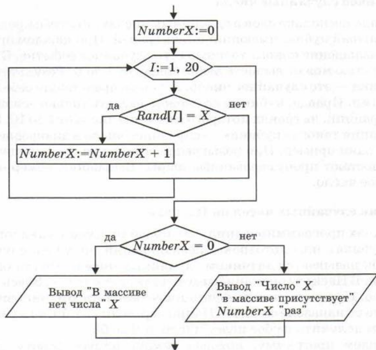
Рис. 2.11. Подсчет вхождений числа в массив
