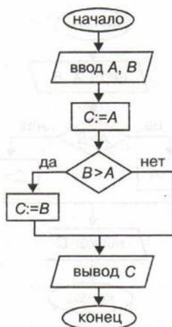
Рис. 2.3. Алгоритм выбора большего из двух значений (с неполным ветвлением)
