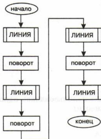
Рис. 1.7. Блок-схема алгоритма «Рамка»
