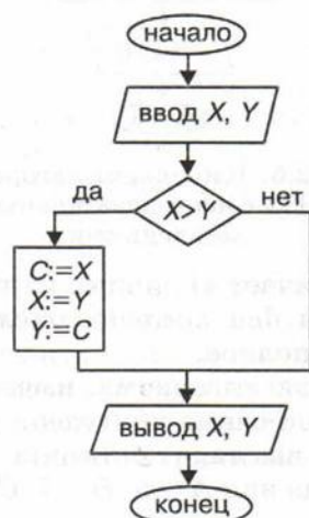
Рис. 2.4. Блок-схема алгоритма упорядочения двух величин
